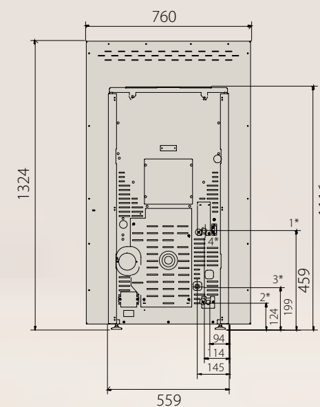
Altea - Selena 15 | 18 Kw
