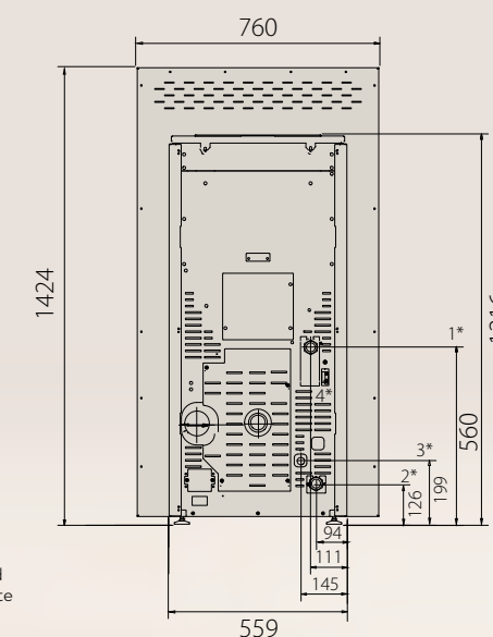
Altea - Selena 27 Kw
